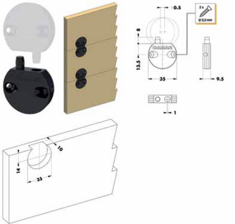
Joint pour paneaux type 814.00.P2.00.01
